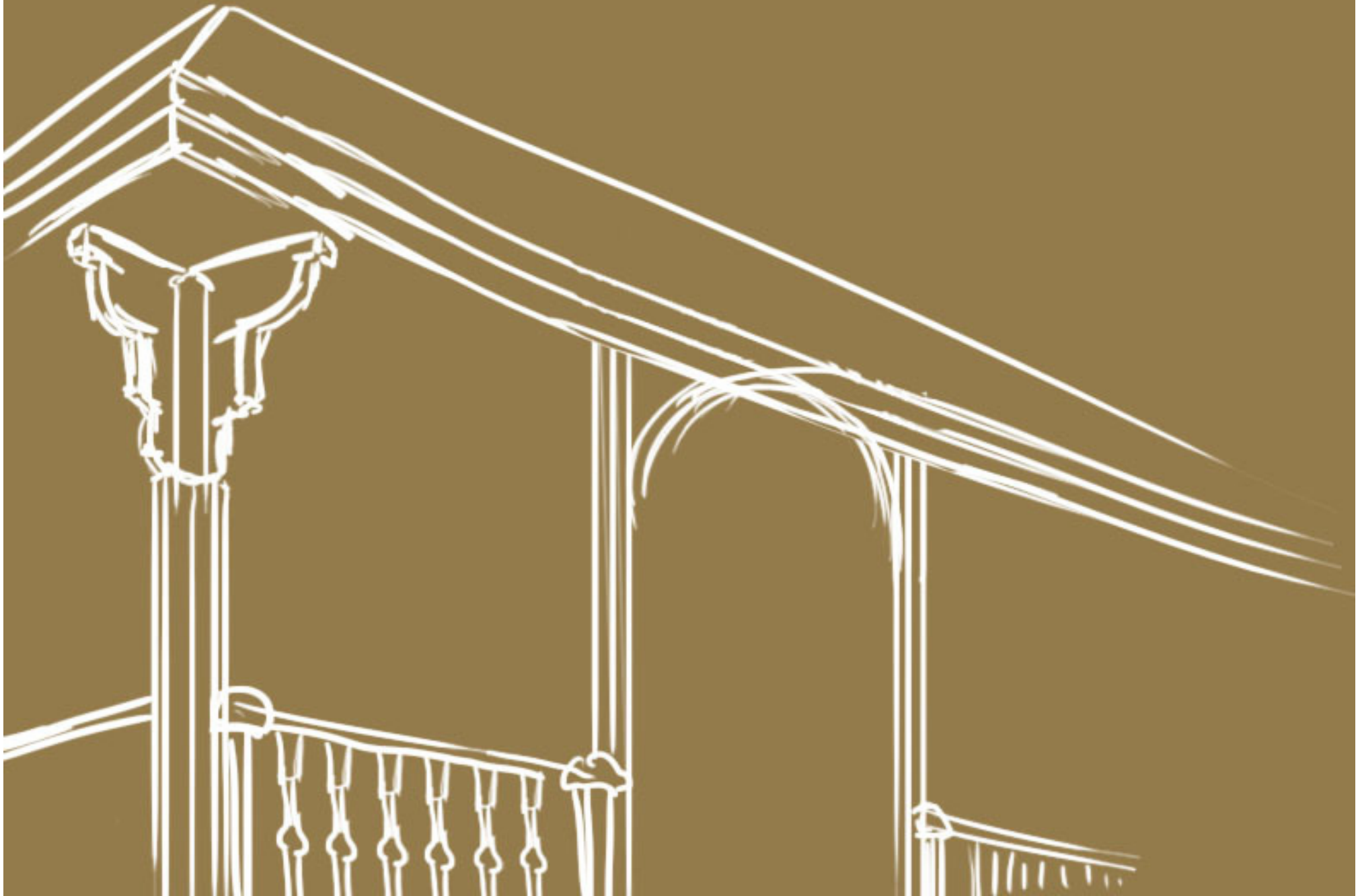
Architecture8.jpg
